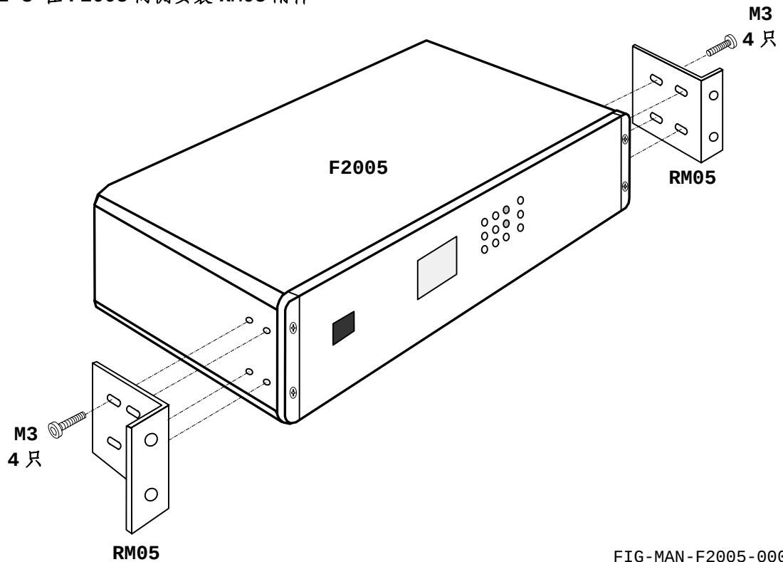
图 2-3 在 F2005 两侧安装 RM05 附件
