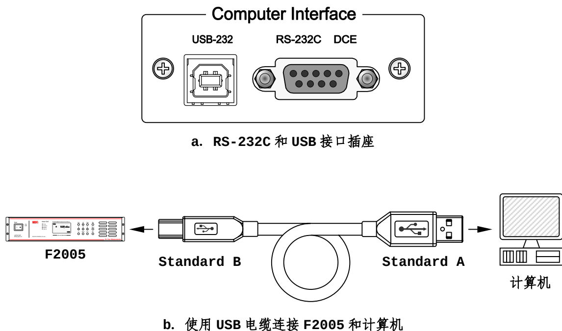
图 2-8 计算机接口连接器以及使用 USB 电缆连接 F2005 和计算机
