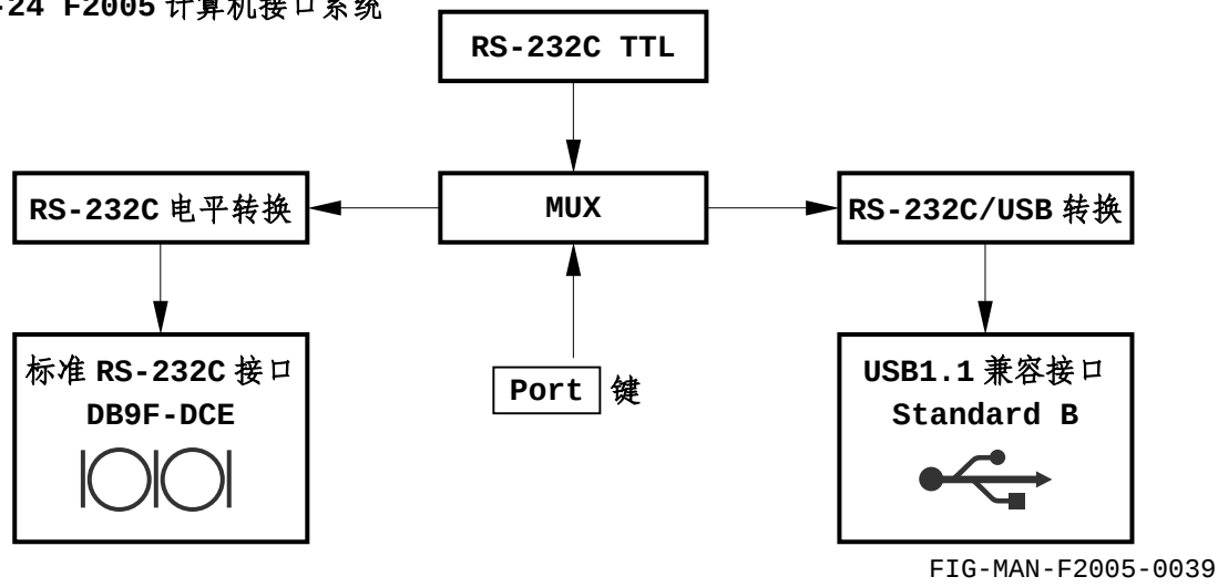
图 3-24 F2005 计算机接口系统
