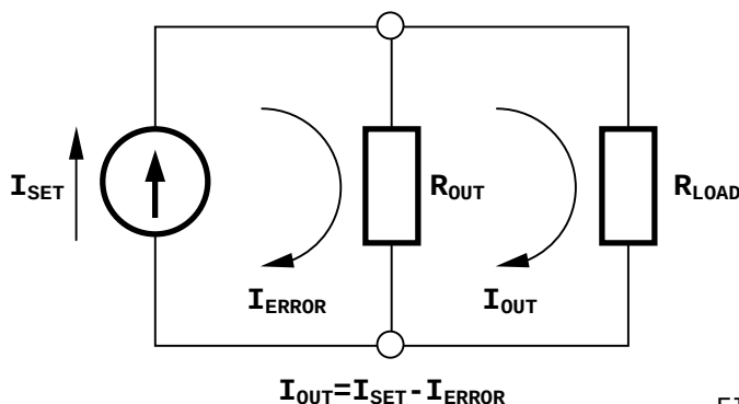
图 3-9 有限输出阻抗 R_{OUT} 造成的分流误差
