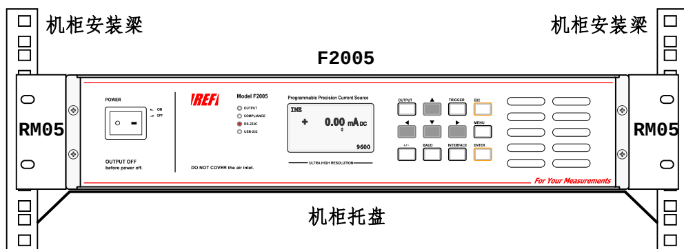
图 2-4 F2005 与机柜的连接安装方法
