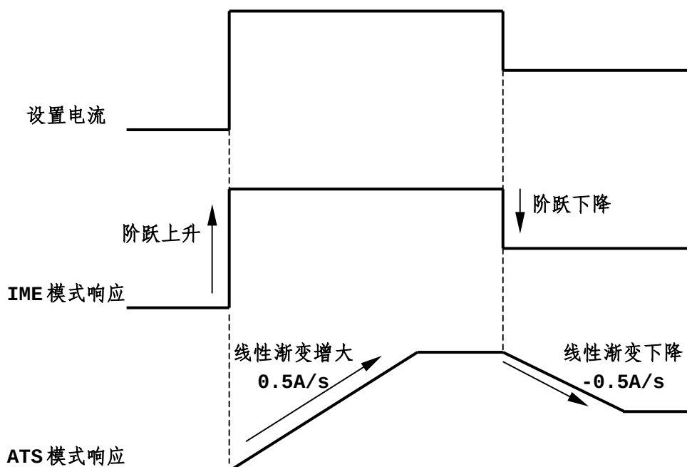
图 3-14 IME 和 ATS 输出响应模式（电流极性为正）
