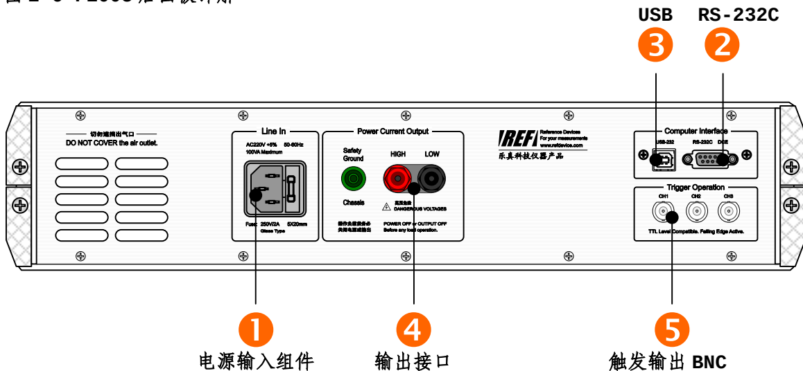
图 2-6 F2005 后面板详解
