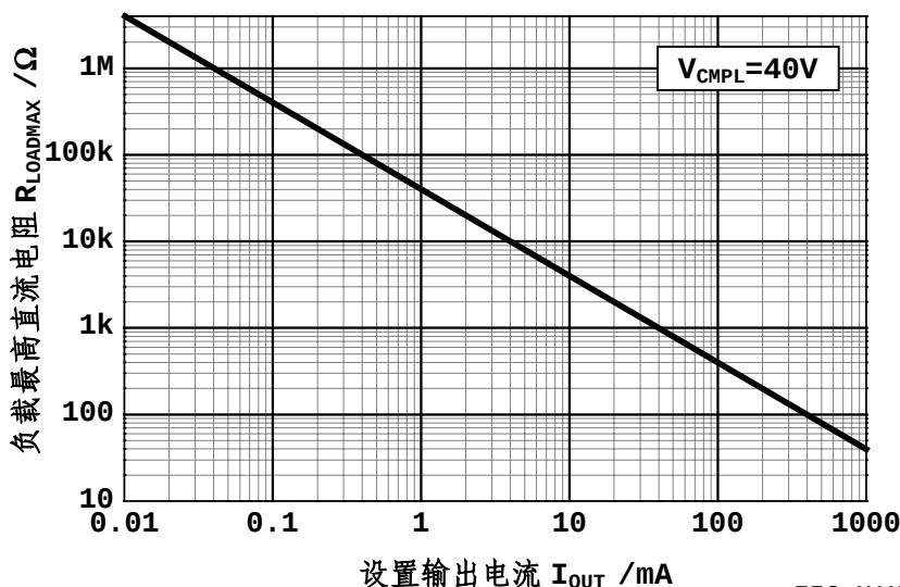
图 3-8 负载最高直流电阻限制
