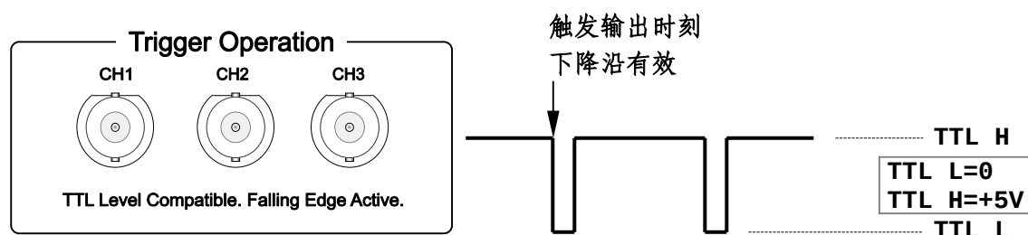
图 2-10 触发输出 BNC 接口和触发电平
