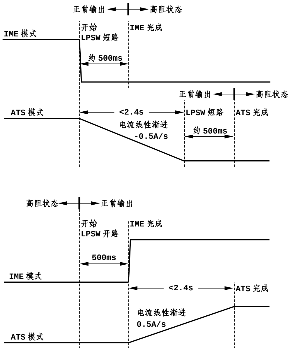
图 3-17 由高阻状态进入正常输出状态时的输出响应
