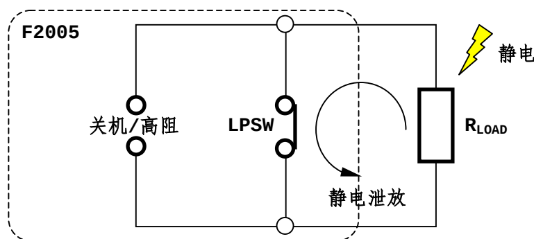
图 3-12 LPSW 提供静电保护
