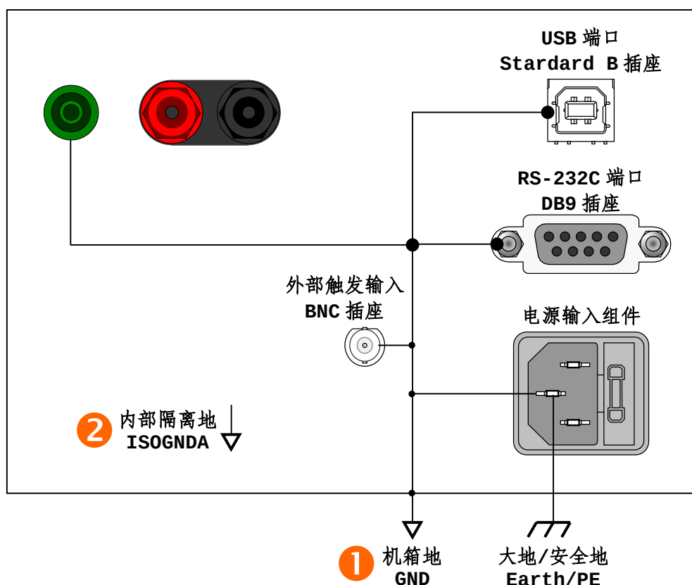
图 3-32 F2005 的接地关系
