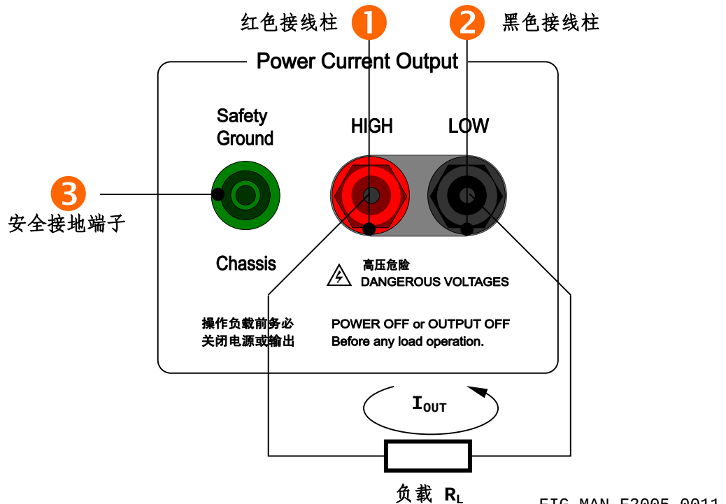
图 2-9 功率电流输出 2 芯接线柱和安全接地端子
