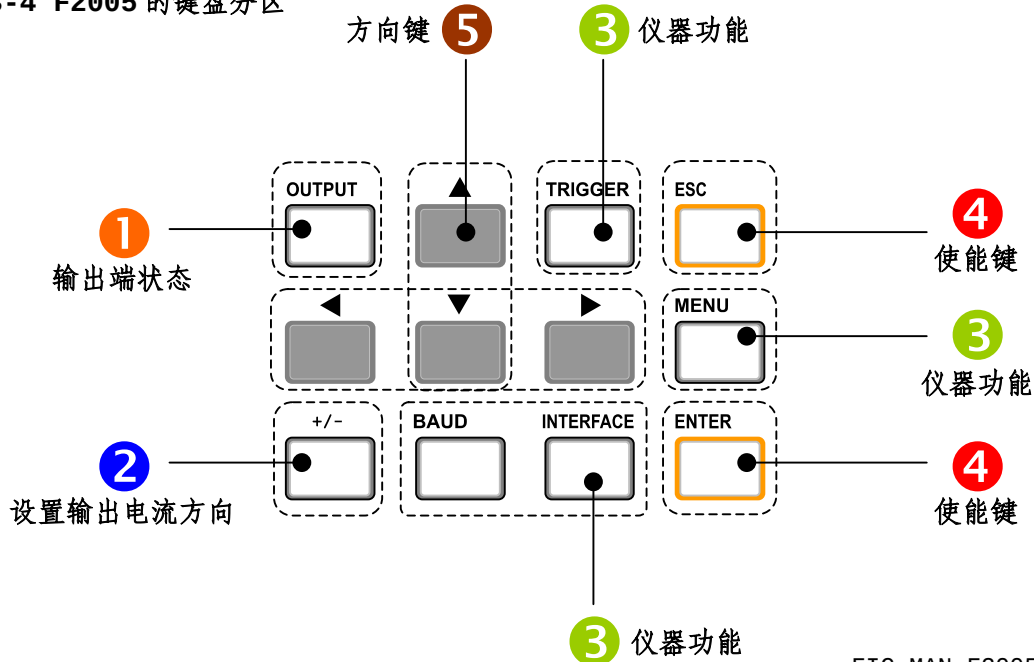
图 3-4 F2005 的键盘分区
