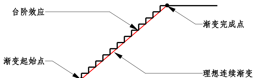
图 3-15 电流线性渐变过程中的台阶效应
