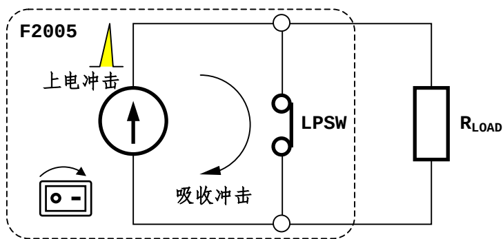
图 3-11 LPSW 保护负载上电安全
