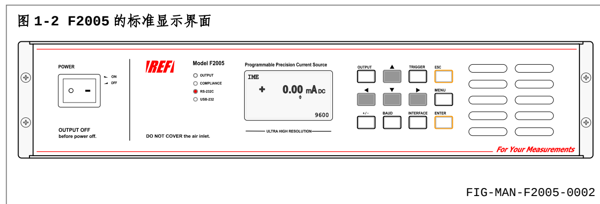
图 1-2 为 F2005 程控精密电流源开机后的标准显示界面。
