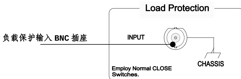
图 2-11 负载保护输入 BNC 接口
