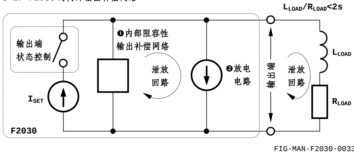
图 3-17 F2030 的内部输出补偿网络
