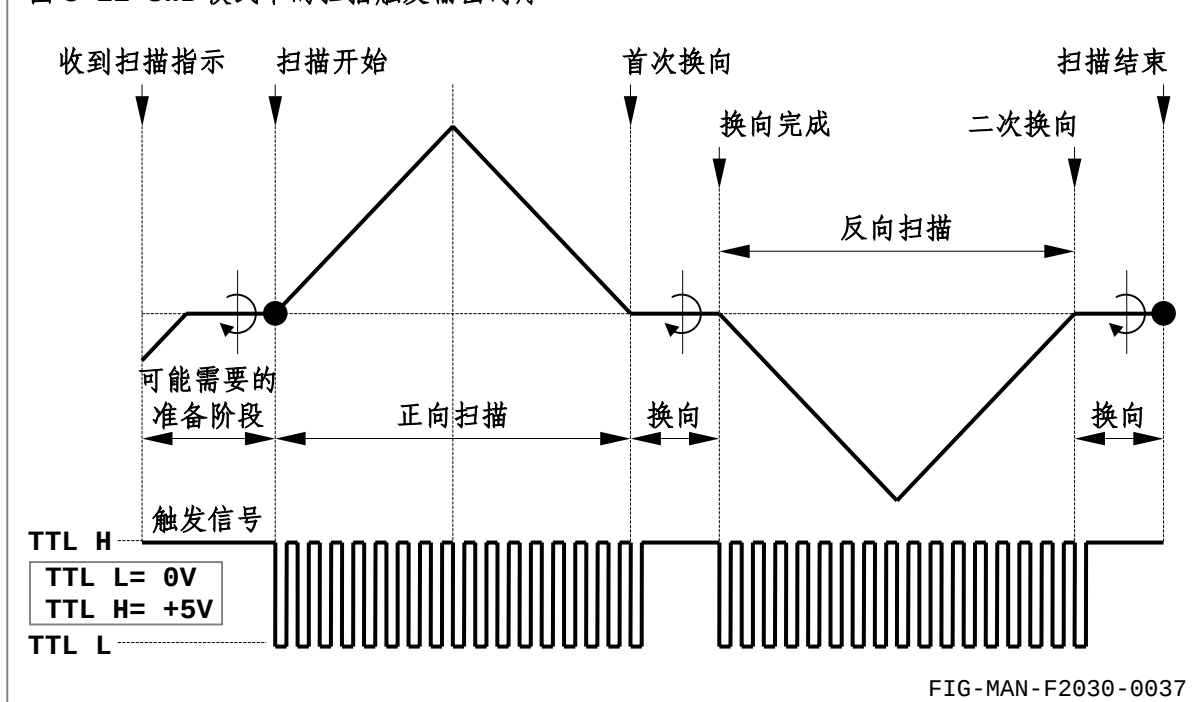
图 3-21 SWB 模式下的扫描触发输出时序
