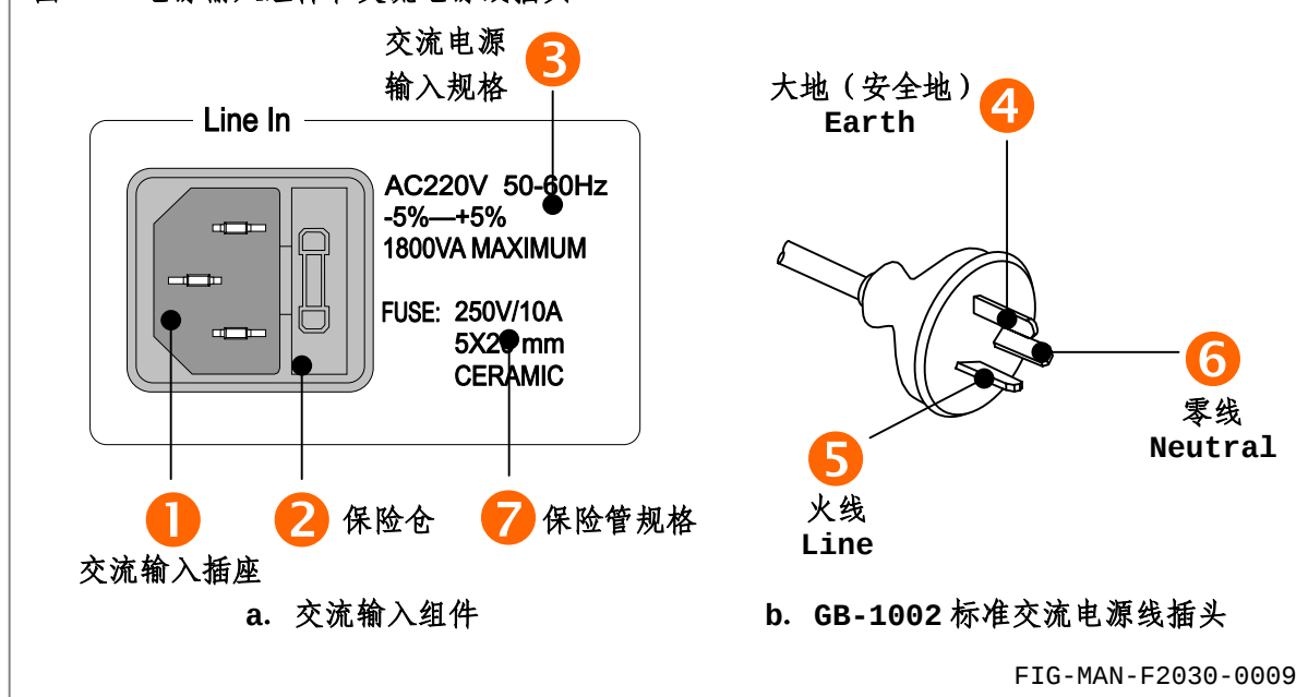
图 2-7 电源输入组件和交流电源线插头
