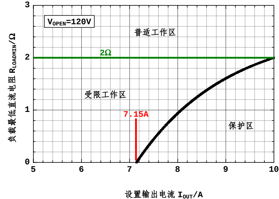
a. 负载最低直流电阻限制 R_{LOADMIN}
