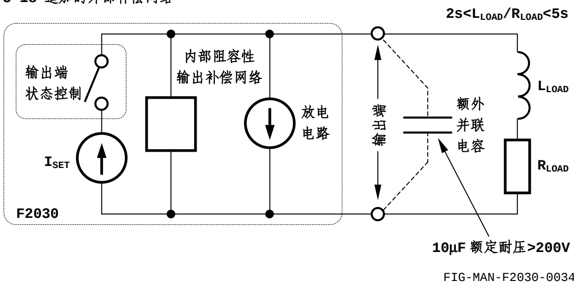
图 3-18 追加的外部补偿网络
