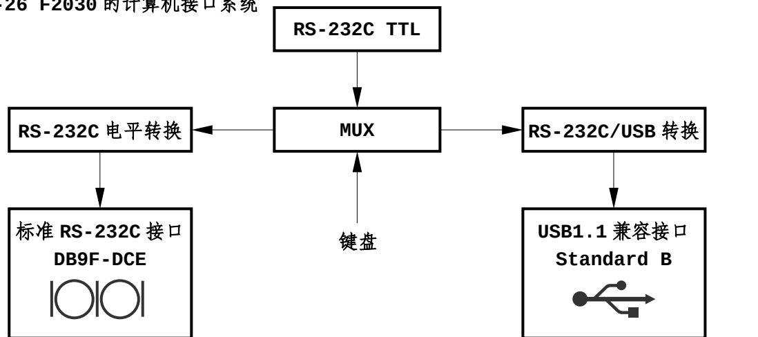
图 3-26 F2030 的计算机接口系统
