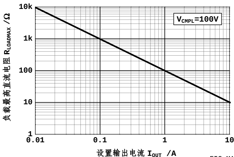
图 3-11 负载最高直流电阻限制
