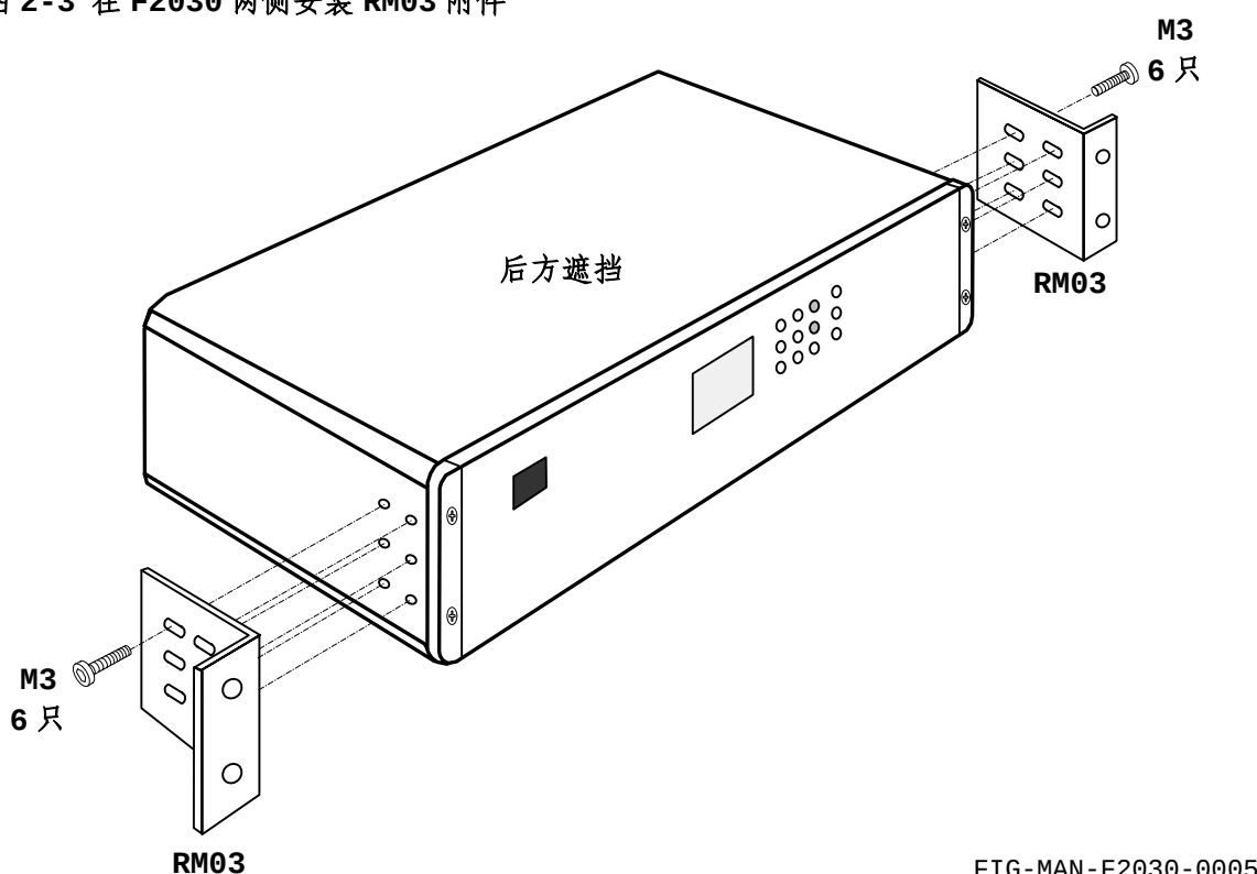
图 2-3 在 F2030 两侧安装 RM03 附件
