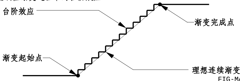
图 3-9 电流线性渐变过程中的台阶效应
