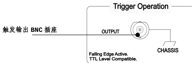
图 2-10 触发输出 BNC 接口
