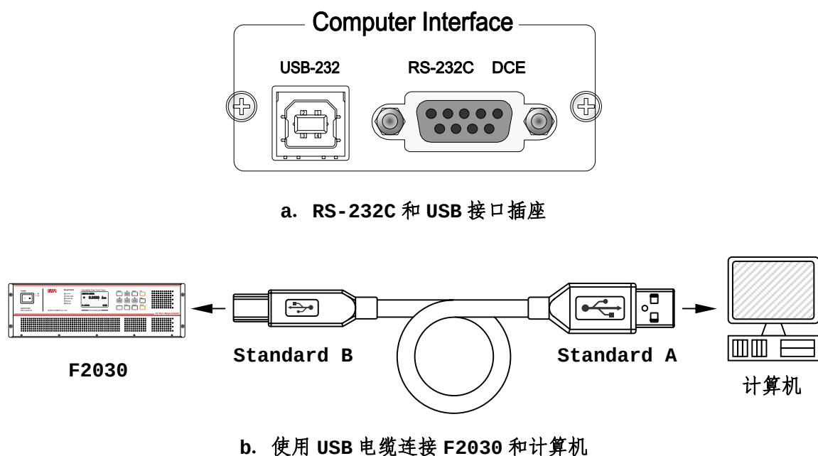
图 2-8 计算机接口连接器以及使用 USB 电缆连接 F2030 和计算机
