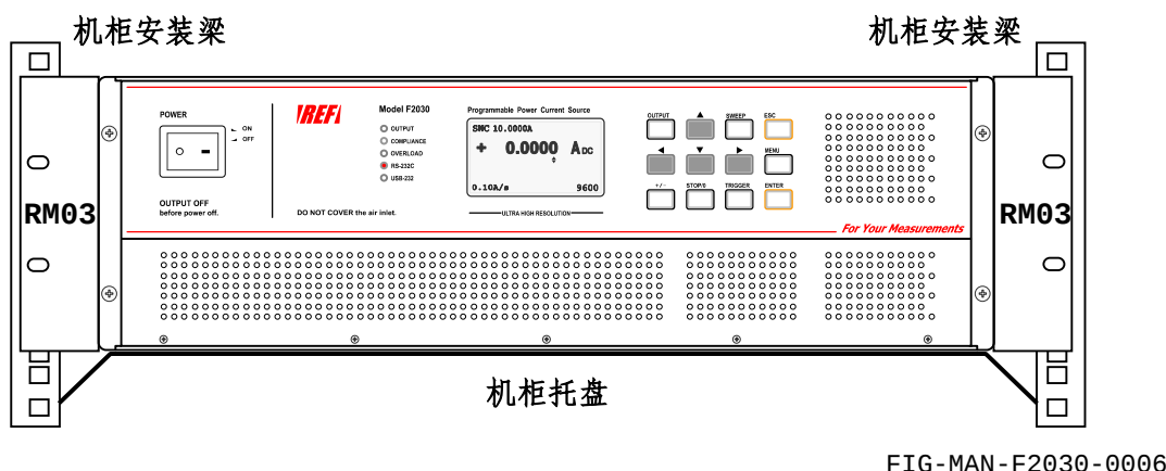
图 2-4 F2030 与机柜的连接安装方法
