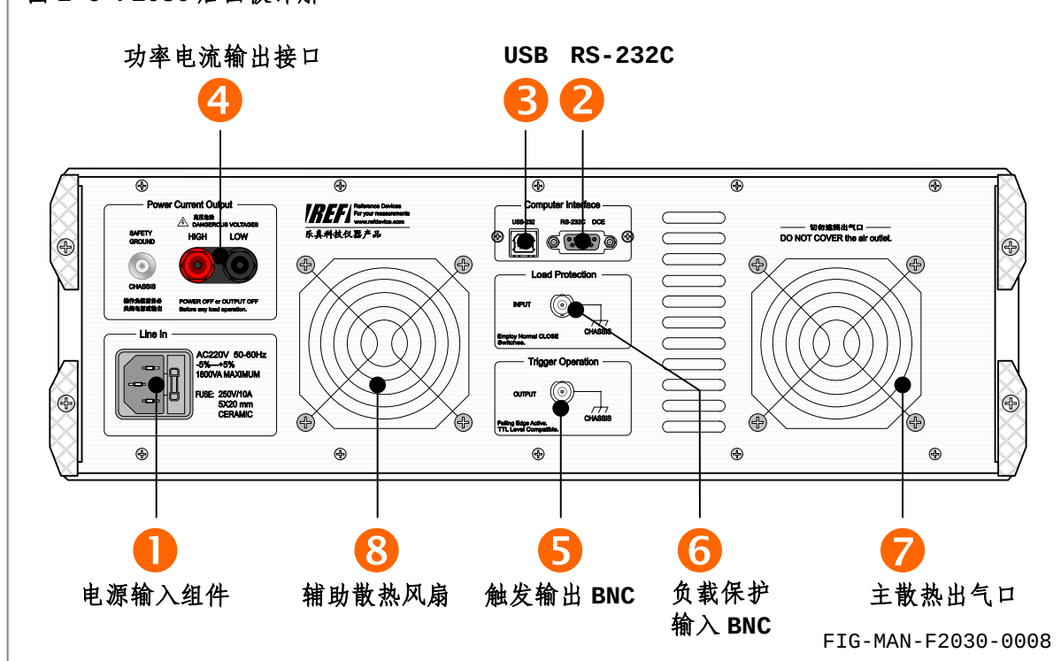
图 2-6 F2030 后面板详解
