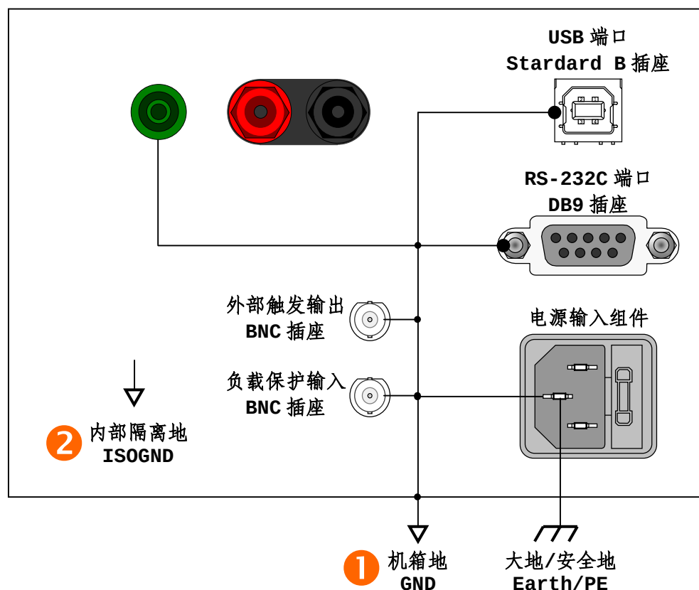
图 3-32 F2030 的接地关系
